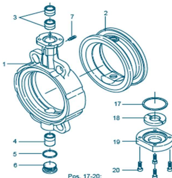
Pos. 17-20: Afdekplaat voor Vlinderklep \geq DN 350
