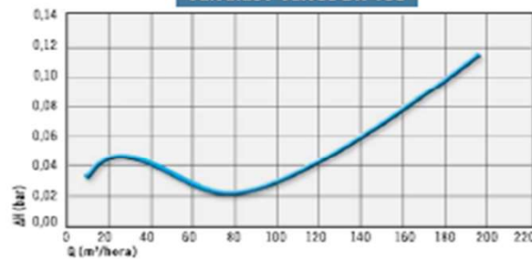
Válvulas / Valves DN 250
