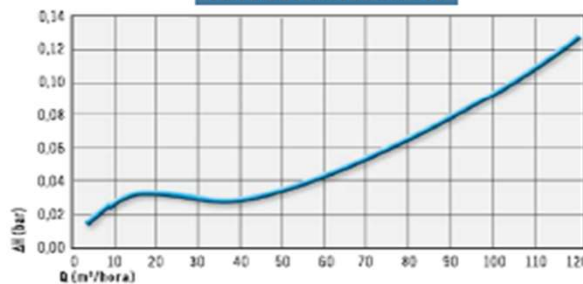
Válvulas / Valves DN 150
